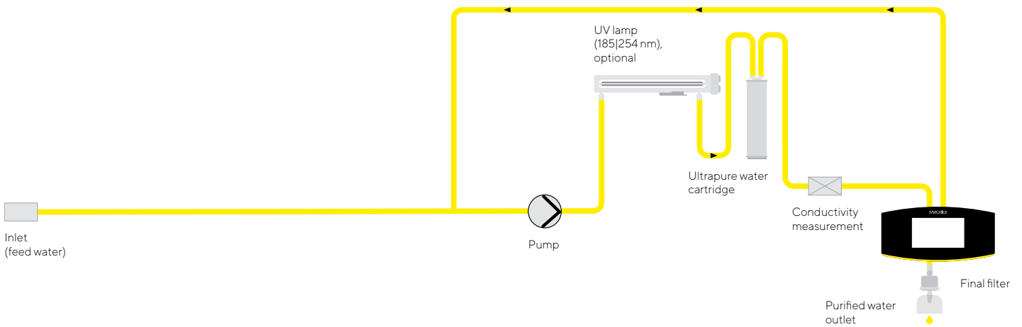
Flow diagram for Arium® Mini Essential
